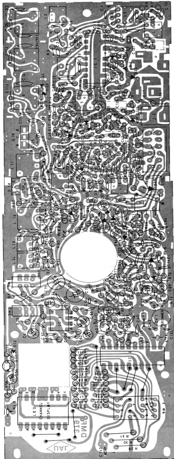
Bestückungsseite
