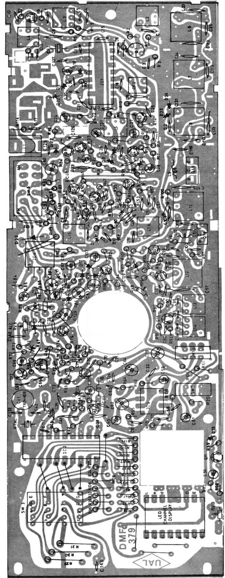
Lötseite
