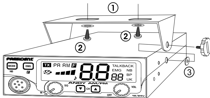
MONTAGESKIZZE
