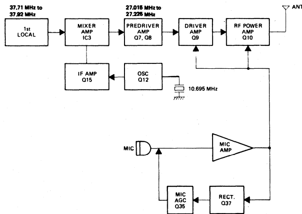
Fig. 10 AM TRANSMITTER
