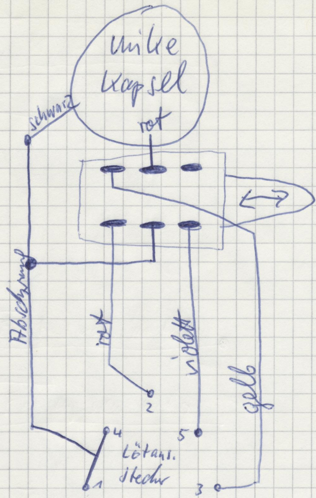
Umbein-Verdrahtung
