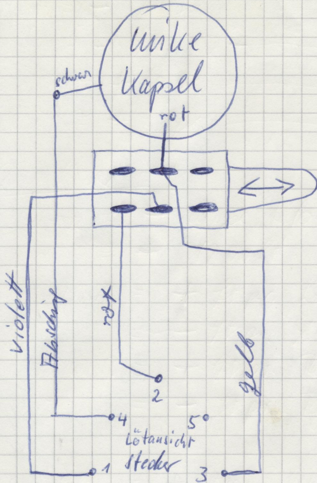
Original-Verdrahtung
