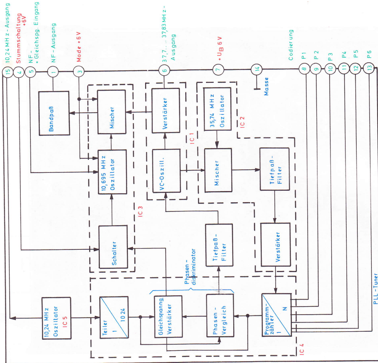
Blockschaltbild PLL-Tuner
