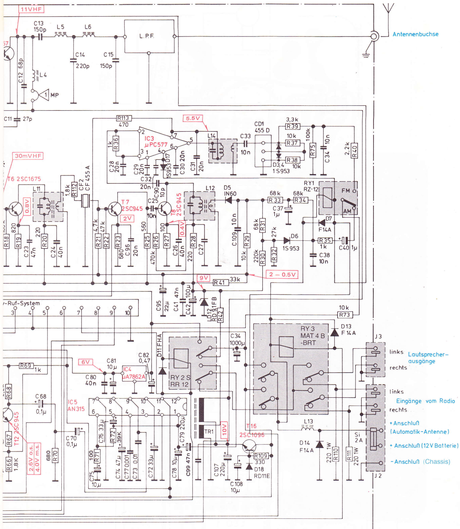
AM/FM-Sender-Empfänger Schaltbild
