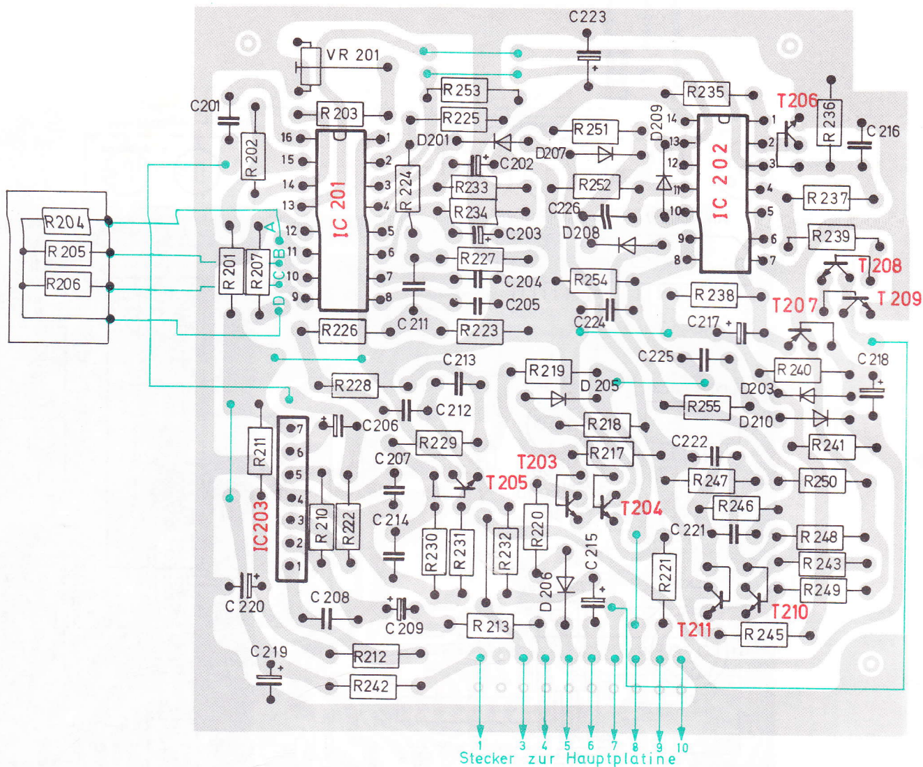
Ansicht von der Lötseite
