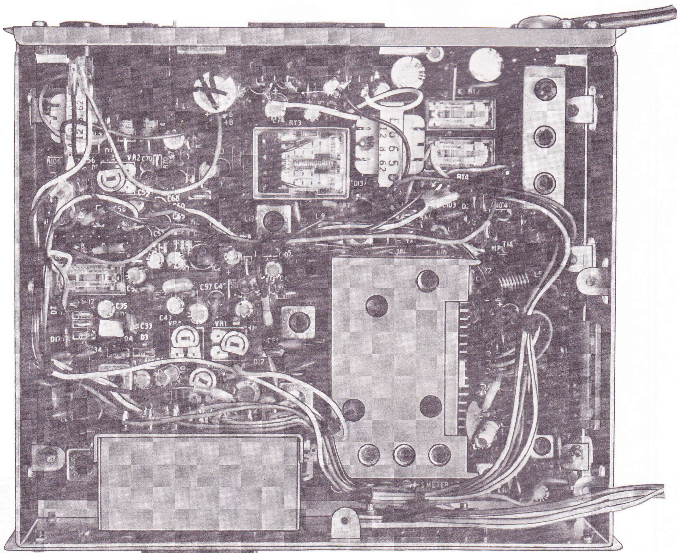
Gerätedraufsicht (bei ausgebautem Selektivruf)
