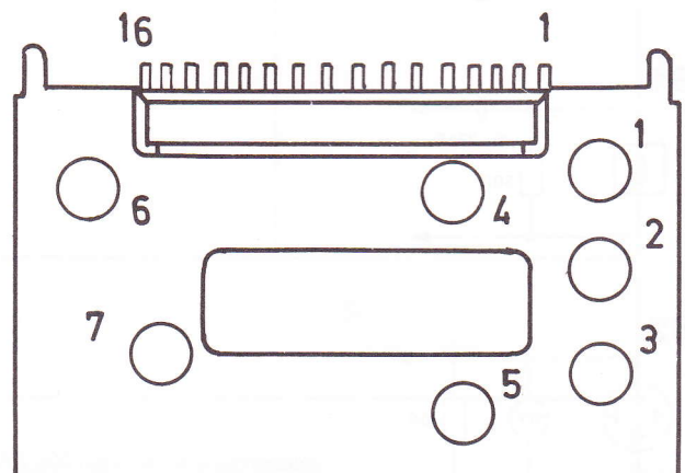
PLL-Tuner: Draufsicht
