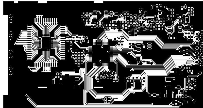
NT 100 LCD PCB REV:0-2 16-JAN-08
