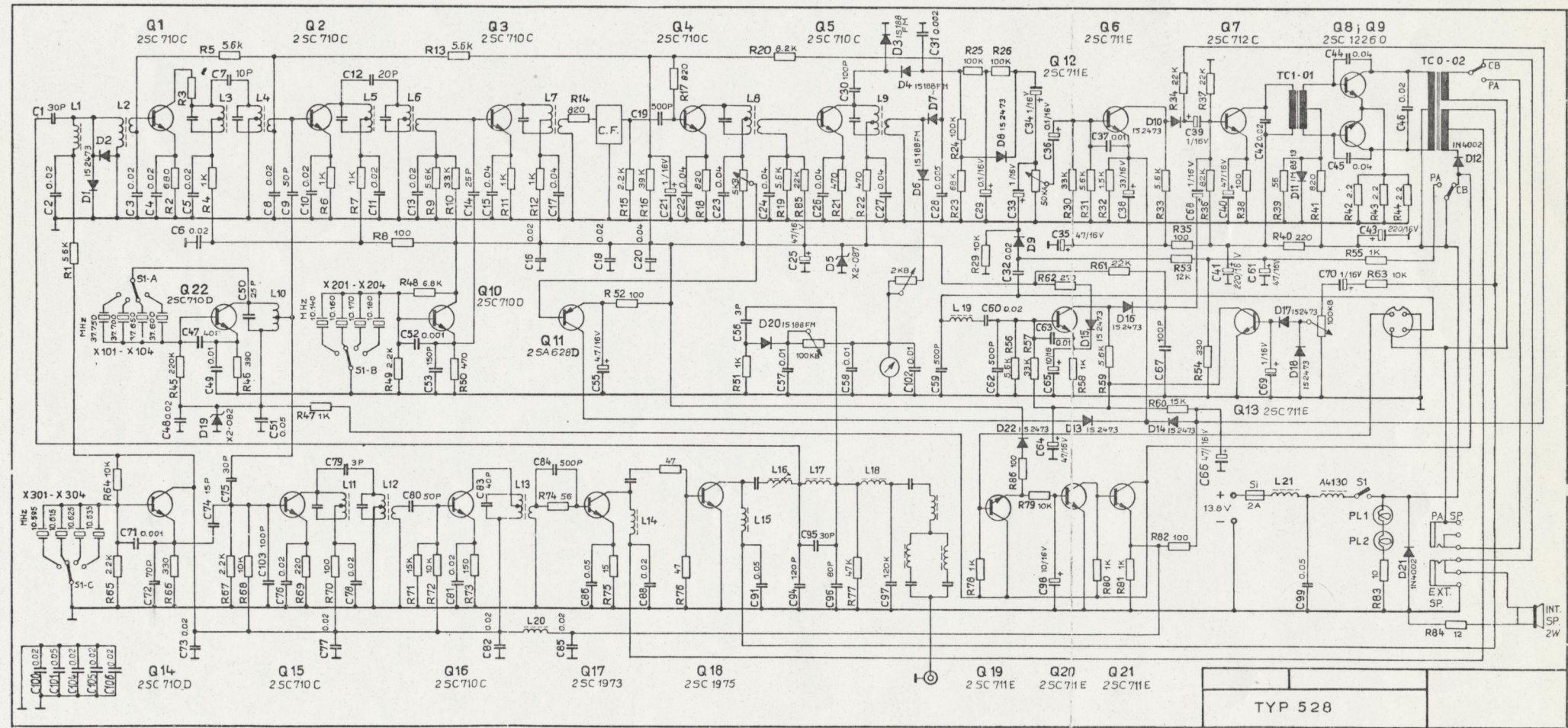
Schaltplan N-Transceiver Basis 528 (ohne Netzteil)
